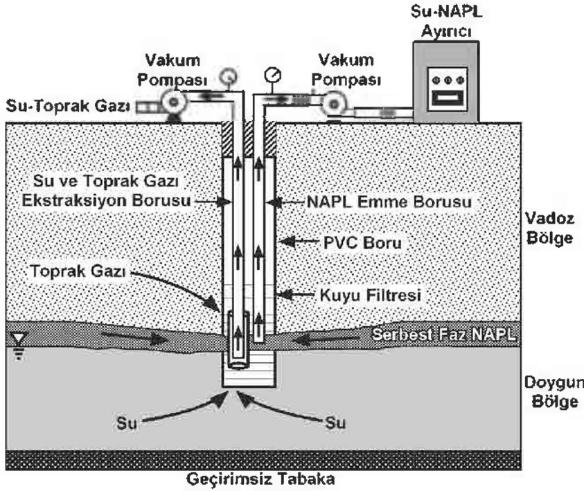
Şekil 5. İkili faz ekstraksiyonu teknolojisinin uygulamasını gösteren şematik çizim (BATTELLE, 1997 ve Place vd., 2003'ten değiştirilerek çizilmiştir)
