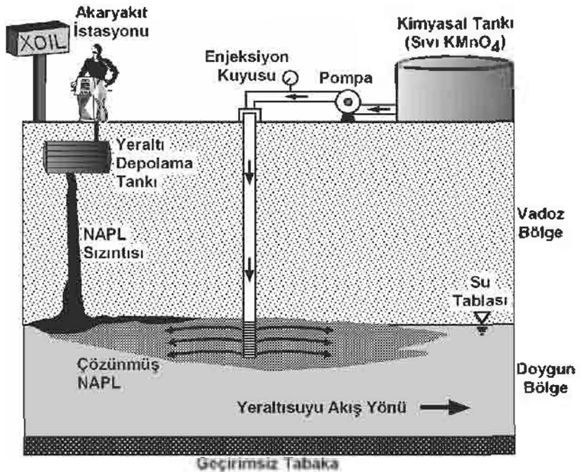
Şekil 6. Kimyasal oksidasyon teknolojisinin uygulamasını gösteren şematik çizim ( www.frtr.gov/matrix2/section4/D01-4-30.html 'den değiştirilerek çizilmiştir)
